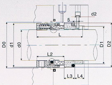
59U型 聚四氟乙烯楔形环
